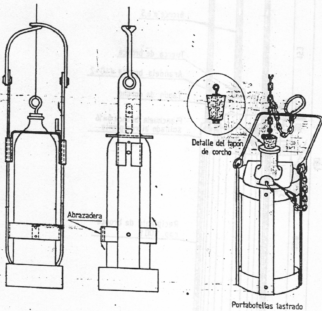
Figura 2 Ejemplos de jaulas portabotellas
