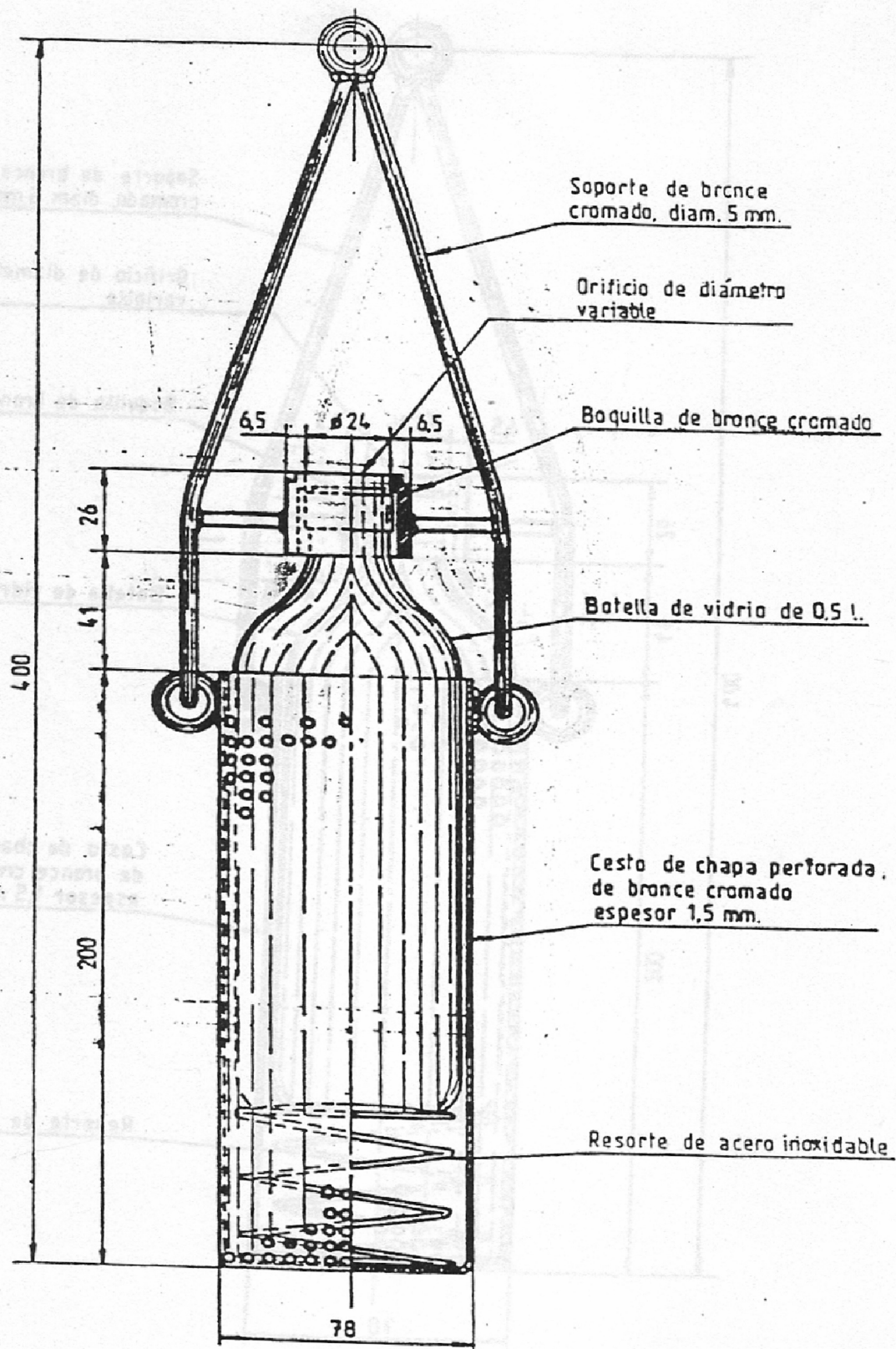
Figura 3 bis Sacamuestra para productos livianos
