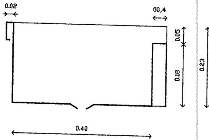
Corte: A-B
